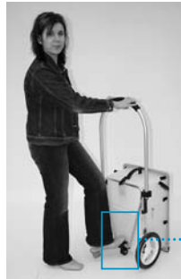
4) Federklemme mit dem Fuss niederdrücken
